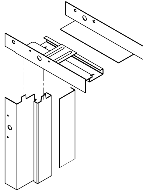
ADJUSTABLE STEEL DOOR FRAME
